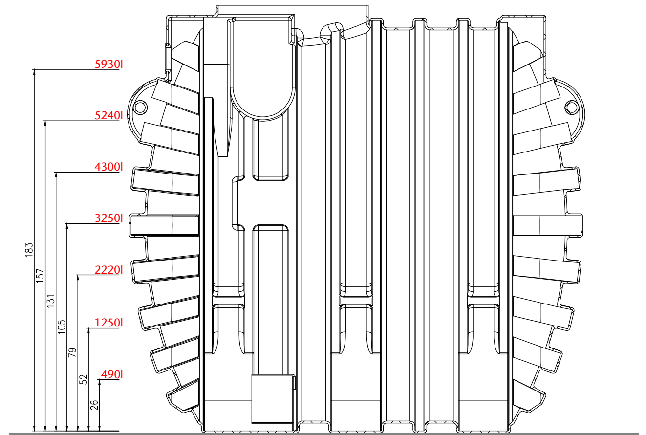
Zisterne 6500l
