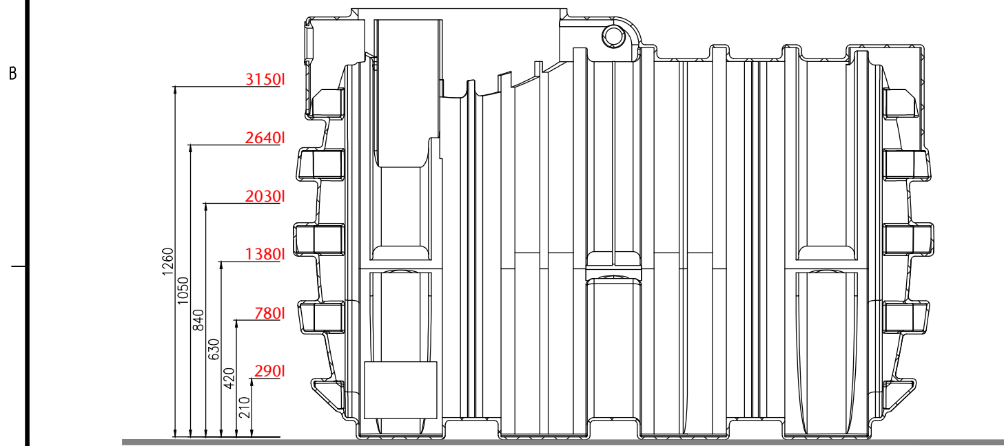
Zisterne 3300l
