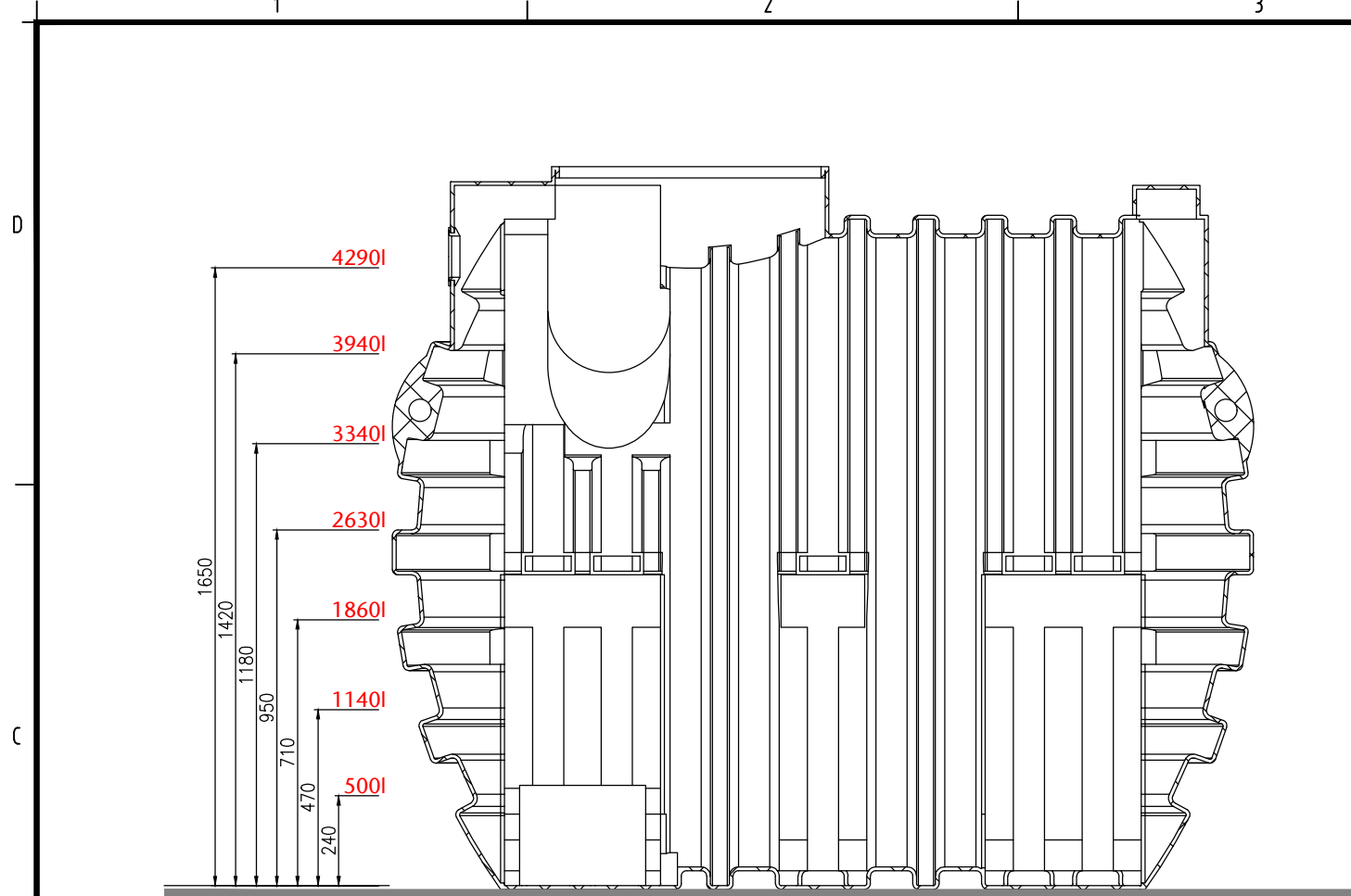
Zisterne 4700l
